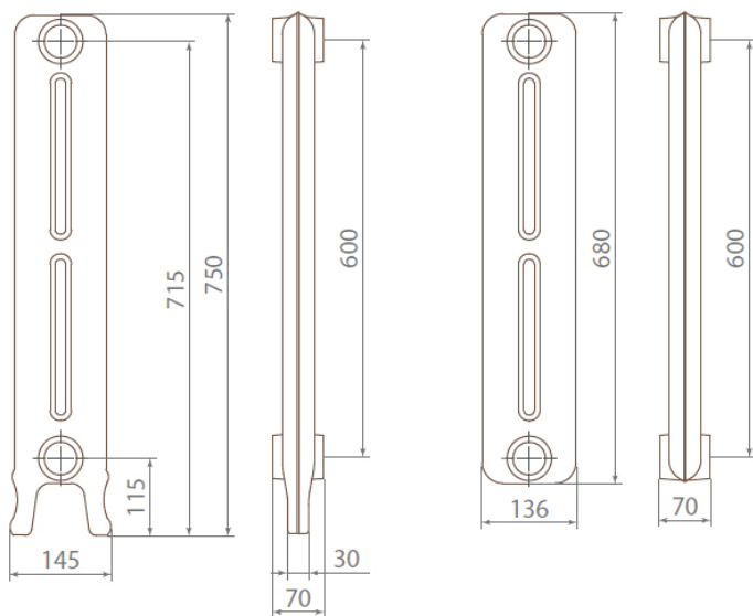
Чертеж секций радиатора EXEMET VENERA 750/600
